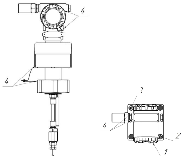
Вид сбоку
