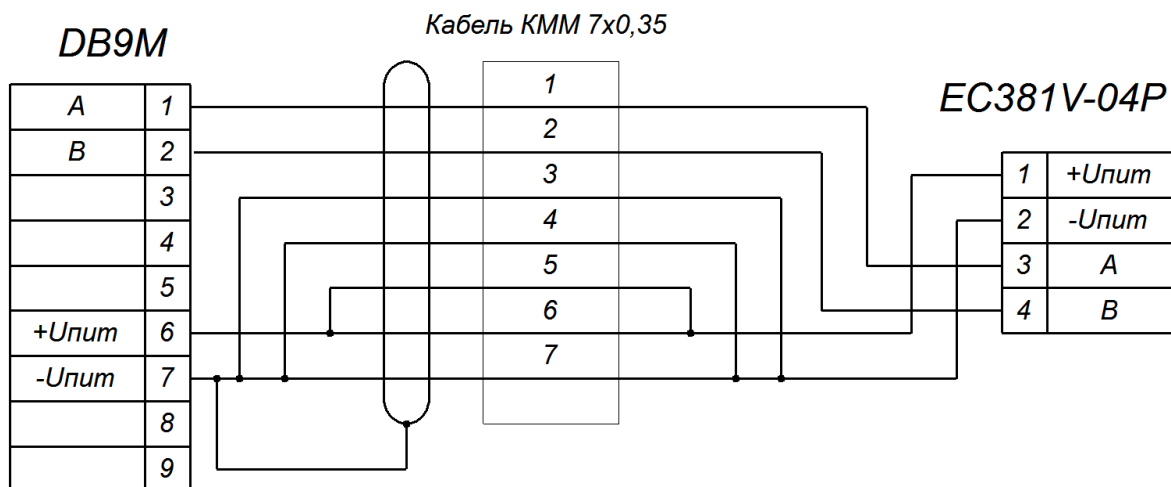
Рисунок В.1 – Схема распайки кабеля КММ 7×0,35
