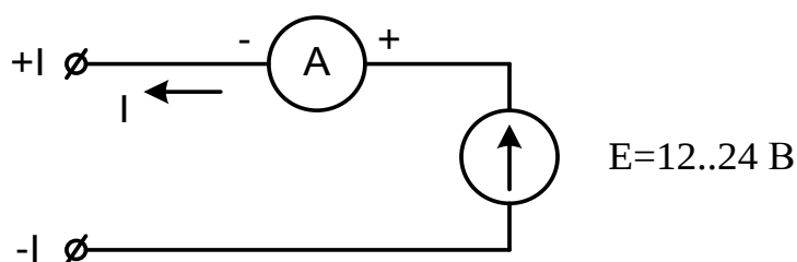
Рисунок 3.4 – Схема подключения приборов для проверки токового выхода
