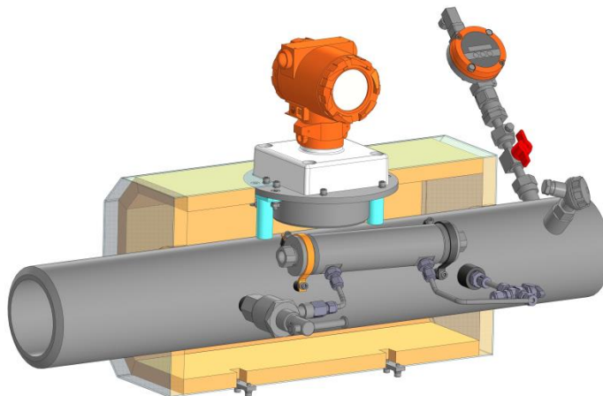
Рисунок 2.10 – Подключение UDM-B по типу «закрытый байпас»
