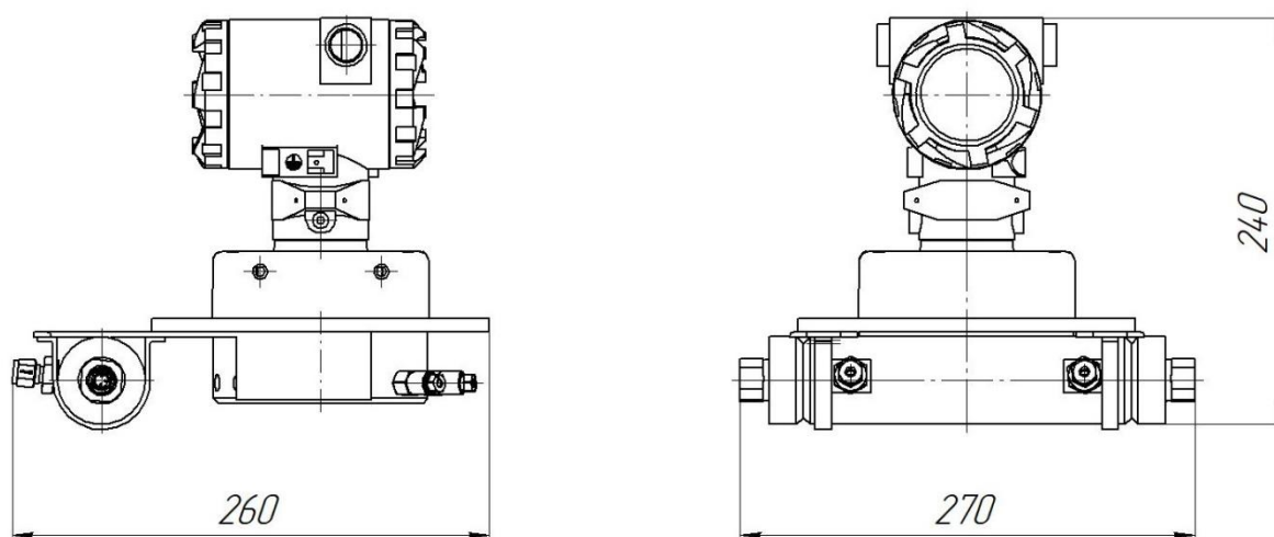
Рисунок Б.2 – Габаритные размеры преобразователя плотности модификации UDM-B
