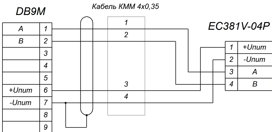
Рисунок В.2 – Схема распайки кабеля КММ 4×0,35
