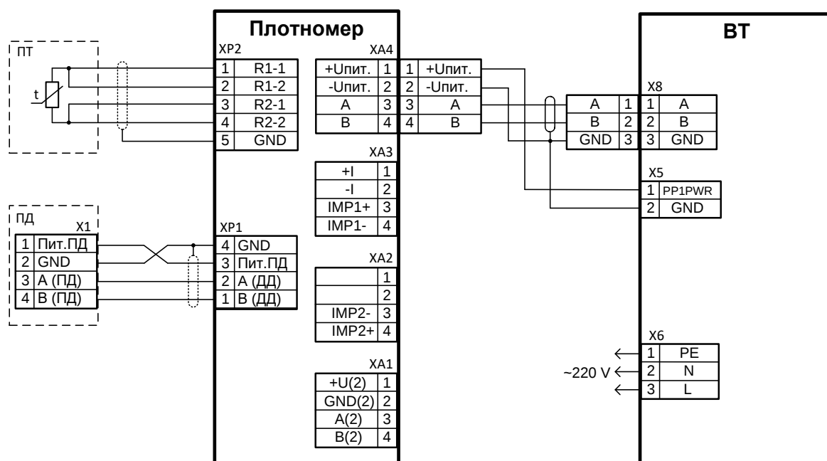
Рисунок В.7 – Схема подключения плотномера к ВТ
