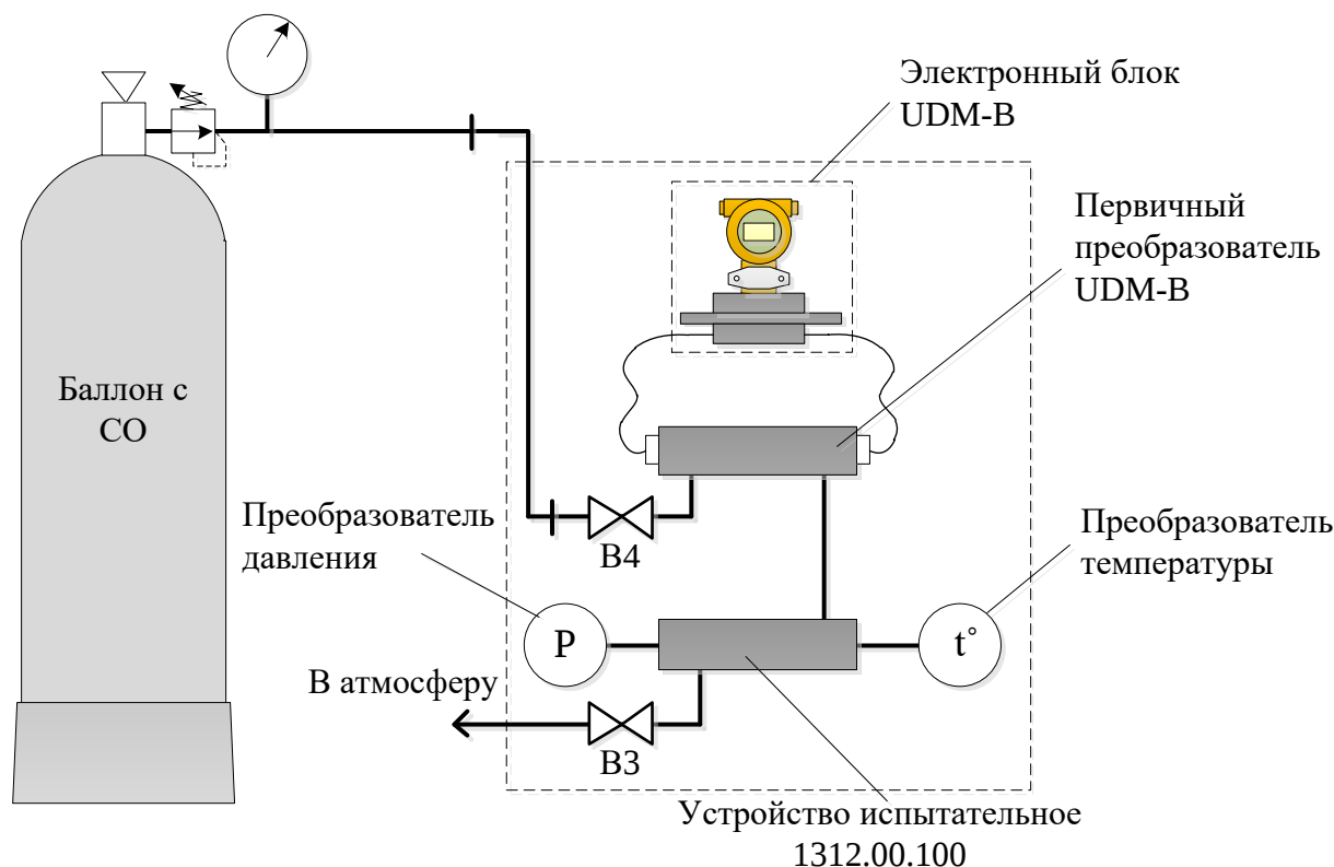
Рисунок 3.3 – Схема подачи СО из баллона в корпус первичного преобразователя модификации UDM-B
