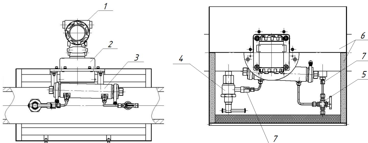
1 – вычислительный модуль плотномера, 2 – измерительный модуль, 3 – измерительная камера, 4 – вентиль пробовотборный, 5 – трехходовой шаровый кран, 6 – полукожухи, 7 – штуцера переходные
