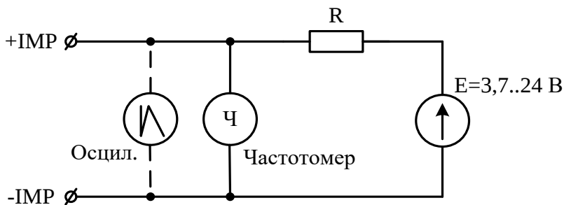
Рисунок 3.5 – Схема подключения приборов для проверки частотных выходов
