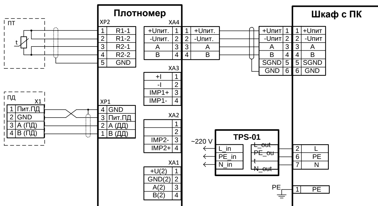
Рисунок В.5 – Схема подключения плотнмера к шкафу с ПК
