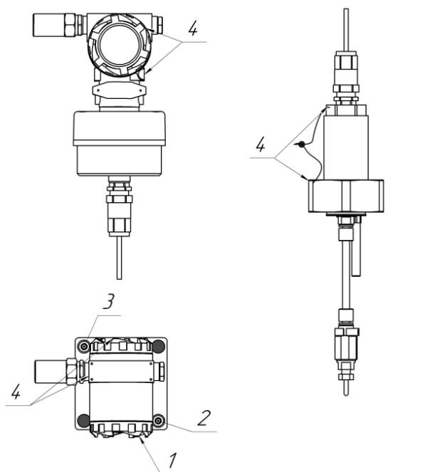
Вид сбоку
