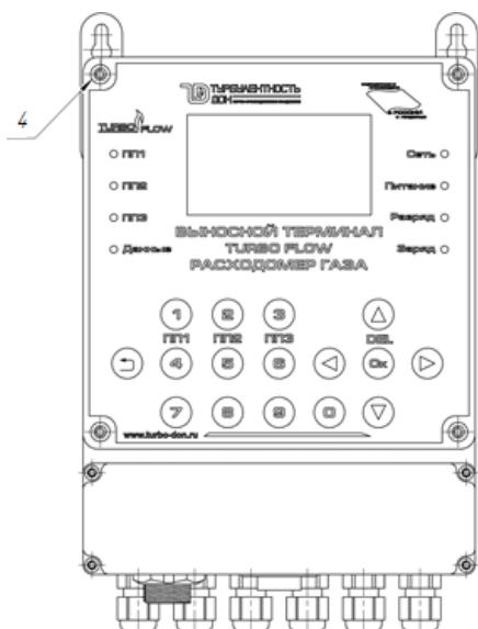
Рисунок 16 - Выносной терминал
