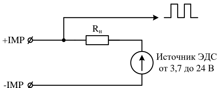
Рисунок 1.10 – Схема подключения к частотным выходам
