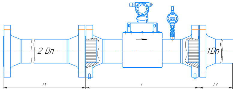
Рисунок Д.48 – Монтаж расходомера класса точности D/D^* \pm 3,0/3,2^* (3,5)^* или \pm 1,5/1,7^* (2,0)^* с УФП С1. Датчик температуры вынесен на трубопровод после расходомера на расстояние не менее 2DN для исполнения корпуса V и С с типом присоединительных фланцев по ГОСТ 33259
