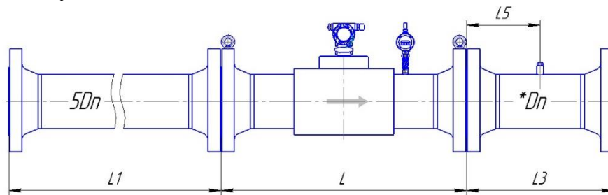
Рисунок Д.19 – Монтаж расходомера класса точности G/G^* \pm 2,0/2,2^* (2,5)^* или \pm 1,0/1,2^* (1,5)^* для исполнения корпуса V по стандарту ASME B16.5-2003
