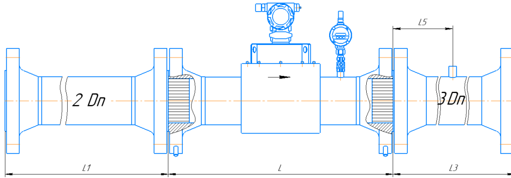
Рисунок Д.41 – Монтаж расходомера класса точности V/V^* \pm 1,0/1,2^* (1,5)^* с УФП С1 для исполнения корпуса V и С с типом присоединительных фланцев по ГОСТ 33259
