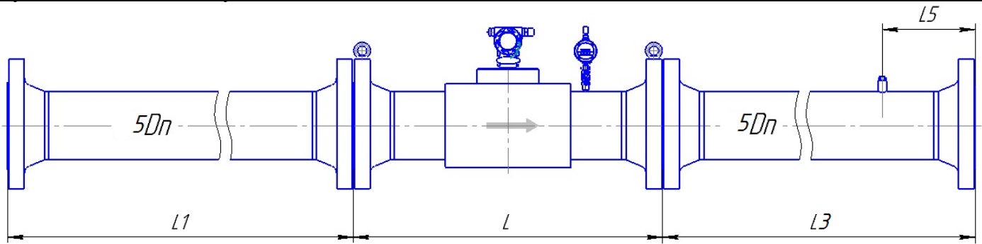
Рисунок Д.11 – Монтаж реверсивного расходомера класса точности D/D^* \pm 3,0/3,2^*(3,5)^* или \pm 1,5/1,7^*(2,0)^* для исполнения корпуса VR и CR с типом присоединительных фланцев по ГОСТ 33259 (* погрешность в зависимости от метода проведения поверки – проливной / имитационный (первичный имитационный и/или периодический имитационный при условии первичной поверки проливным методом; в скобках указана погрешность при периодическом имитационном методе, при условии проведения первичной поверки имитационным методом;))
