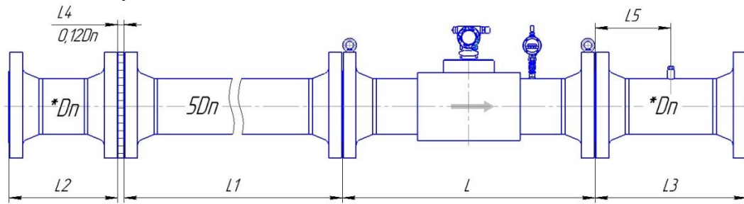
Рисунок Д.16 – Монтаж расходомера с УФП укороченной длины классов точности А ±0,5 и Б ±0,5 для исполнения корпуса V по стандарту ASME B16.5-2003 (при условии калибровки в сборе)
