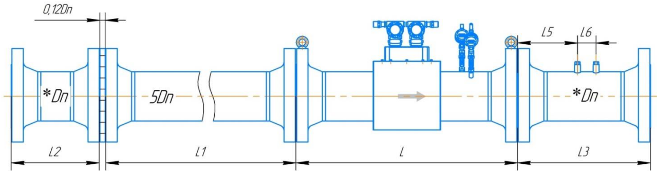
Рисунок Д.37 – Монтаж расходомера с УФП класса точности V/V^* \pm 1,0/1,2^* (1,5)^* для исполнения с дублированием по стандарту ASME B16.5-2003
