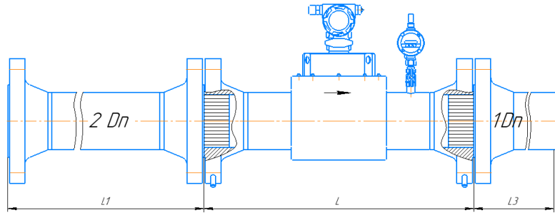
Рисунок Д.47 – Монтаж расходомера класса точности \Gamma/\Gamma^* \pm 2,0/2,2^* (2,5)^* или \pm 1,0/1,2^* (1,5)^* с УФП С1. Датчик температуры вынесен на трубопровод после расходомера на расстояние не менее 2DN для исполнения корпуса V и С с типом присоединительных фланцев по ГОСТ 33259
