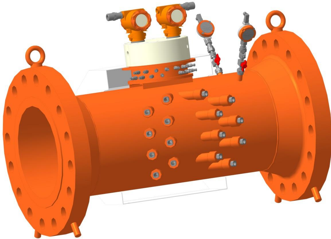
Рисунок Б.11 - Расходомер - счетчик газа ультразвуковой исполнение с дублированием dA
