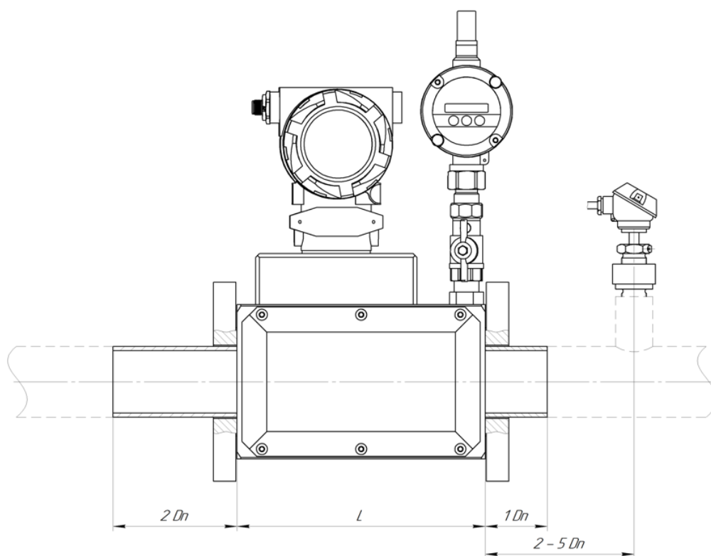
Рисунок Д.52 – Монтаж расходомера класса точности \Gamma/\Gamma^* \pm 2,0/2,2^* (2,5)^* или \pm 1,0/1,2^* (1,5)^* с УФП С1 для исполнения корпуса С с ПУ под приварку
