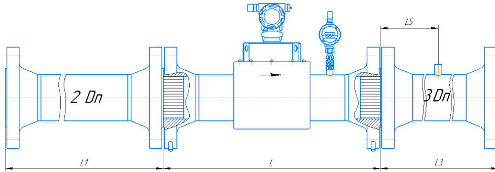
Рисунок Д.43 – Монтаж расходомера класса точности D/D^* \pm 3,0/3,2^*(3,5)^* или \pm 1,5/1,7^*(2,0)^* с УФП С1 для исполнения корпуса V и С с типом присоединительных фланцев по ГОСТ 33259
