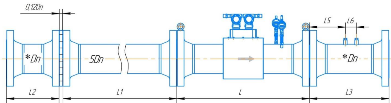
Рисунок Д.34 – Монтаж расходомера с УФП укороченной длины классов точности А ±0,5 и Б ±0,5 для исполнения с дублированием по стандарту ASME B16.5-2003 (при условии калибровки в сборе)
