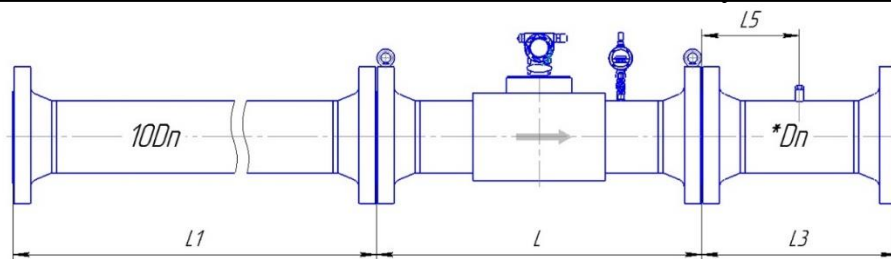
Рисунок Д.4 – Монтаж расходомера класса точности V/B^* \pm 1,0/1,2^* (1,5)^* для исполнения корпуса V и C с типом присоединительных фланцев по ГОСТ 33259
