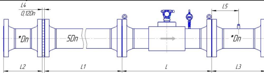
Рисунок Д.5 – Монтаж расходомера с УФП класса точности В/В*±1,0/1,2* (1,5)* для исполнения корпуса V и С с типом присоединительных фланцев по ГОСТ 33259
