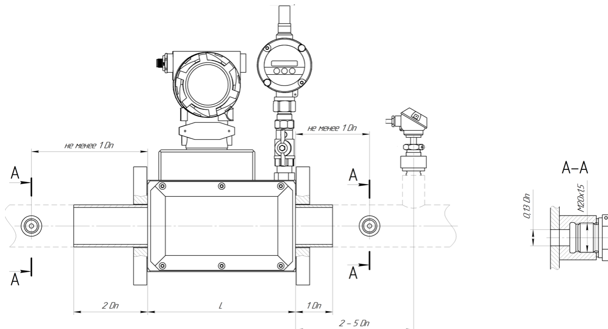
Рисунок Д.51 – Монтаж расходомера класса точности \Gamma/\Gamma^* \pm 2,0/2,2^* (2,5)^* или \pm 1,0/1,2^* (1,5)^* с УФП С1 для исполнения корпуса С с ПУ под приварку с патрубками для эндоскопа Место ввода эндоскопа предусмотрено опломбировать в соответствии с рисунком Е.6 (Установка патрубка для эндоскопа: Ду отверстия не более 0,13 D_n , расстояние от корпуса УЗПП до патрубка ввода эндоскопа - не менее 1 D_n )
