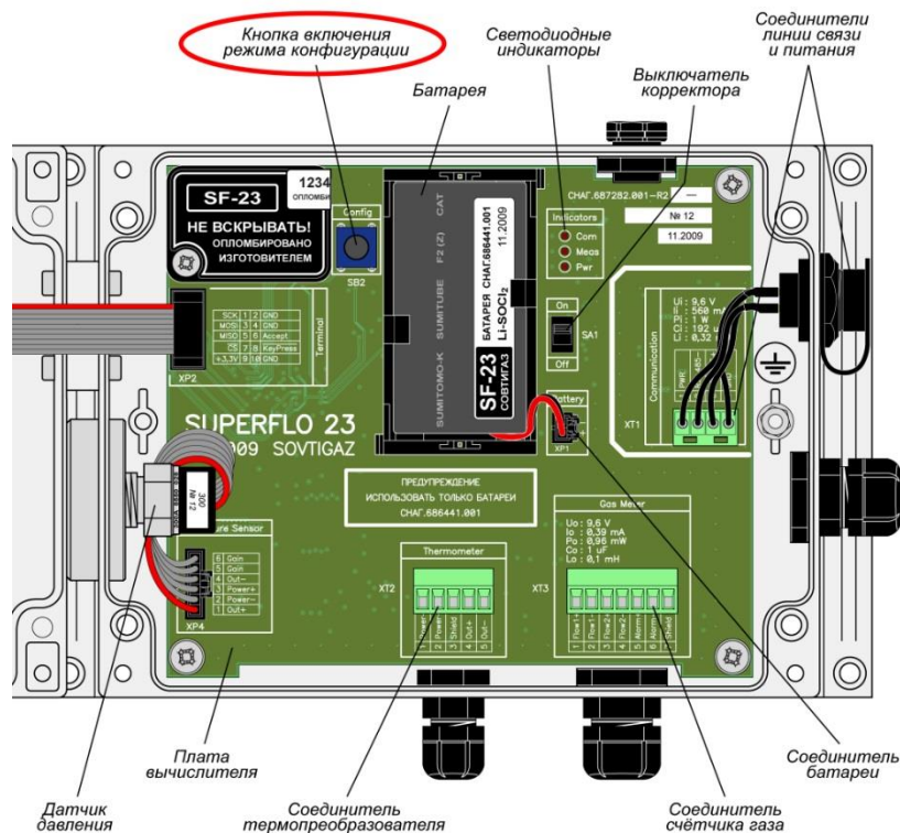
Рисунок 2.71 – Плата корректора
