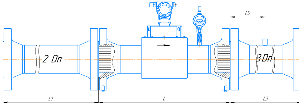
Рисунок Д.42 – Монтаж расходомера класса точности G/G^* \pm 2,0/2,2^* (2,5)^* или \pm 1,0/1,2^* (1,5)^* с УФП С1 для исполнения корпуса V и С с типом присоединительных фланцев по ГОСТ 33259
