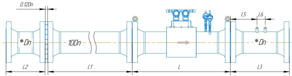
Рисунок Д.33 – Монтаж расходомера с УФП классов точности А/А*±0,5/0,7*(0,7)* и Б/Б ±0,5/0,7*(0,7)* для исполнения с дублированием по стандарту ASME В16.5-2003
