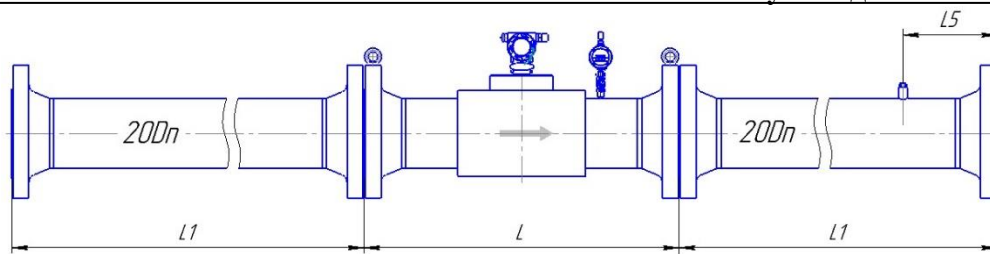
Рисунок Д.21 – Монтаж реверсивного расходомера классов точности А/А*±0,5/0,7*(0,7)* и Б/Б ±0,5/0,7*(0,7)* для исполнения корпуса VR по стандарту ASME B16.5-2003
