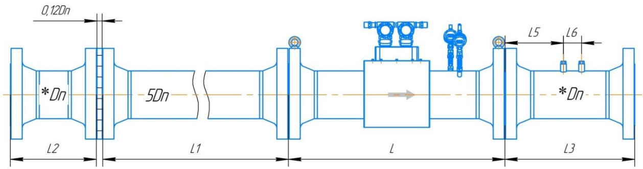
Рисунок Д.27 – Монтаж расходомера с УФП укороченной длины классов точности А ±0,5 и Б ±0,5 для исполнения с дублированием с типом присоединительных фланцев по ГОСТ 33259 (при условии калибровки в сборе)
