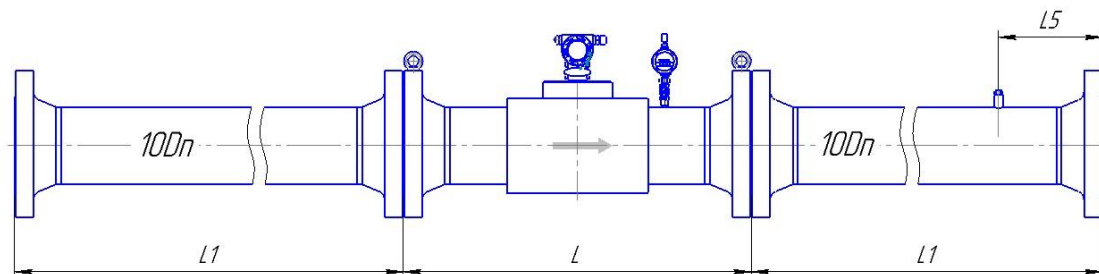
Рисунок Д.22 – Монтаж реверсивного расходомера классов точности V/V^* \pm 1,0/1,2^* (1,5)^* для исполнения корпуса VR по стандарту ASME B16.5-2003
