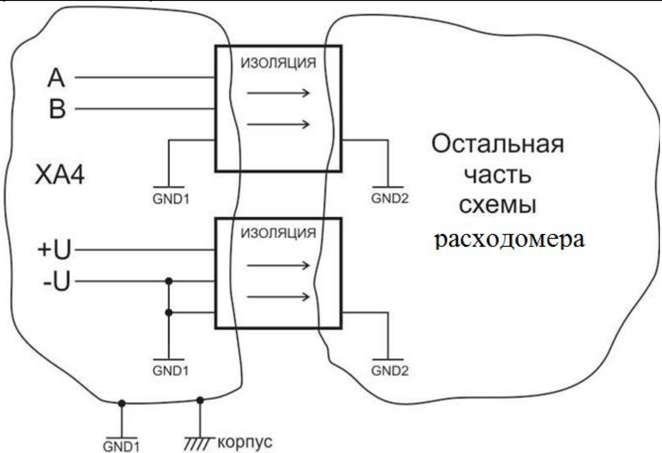
Рисунок 1.15 – Изоляция основного интерфейса RS-485
