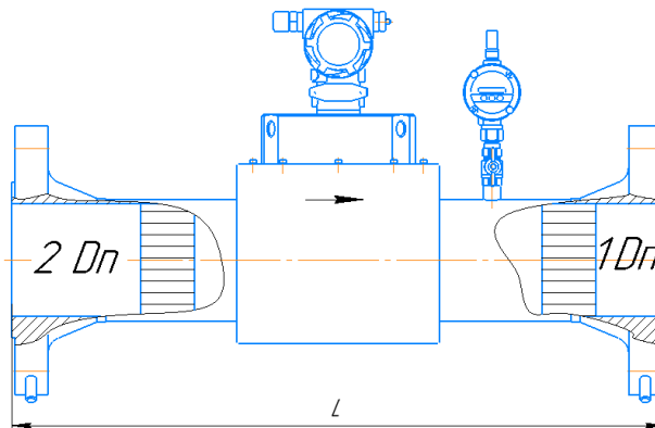
Рисунок Д.44 – Монтаж расходомера класса точности \Gamma/\Gamma^* \pm 2,0/2,2^*(2,5)^* или \pm 1,0/1,2^*(1,5)^* с УФП С1 и прямолинейными участками установленными в едином корпусе расходомера. Датчик температуры вынесен на трубопровод после расходомера на расстояние не менее 2DN для исполнения корпуса V и С с типом присоединительных фланцев по ГОСТ 33259
